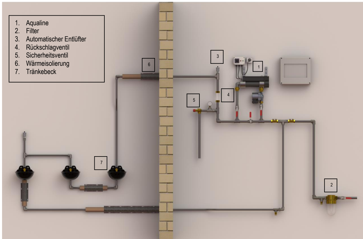
Schema der hydraulischen Installation (Beispiel)
