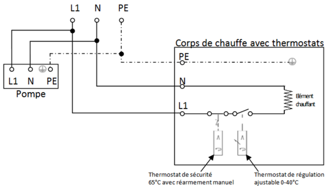
Aqualine avec boîtier de contrôle
