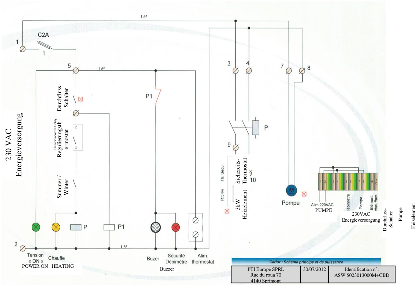
Bild innerhalb des digitalen Kontrollkastens
