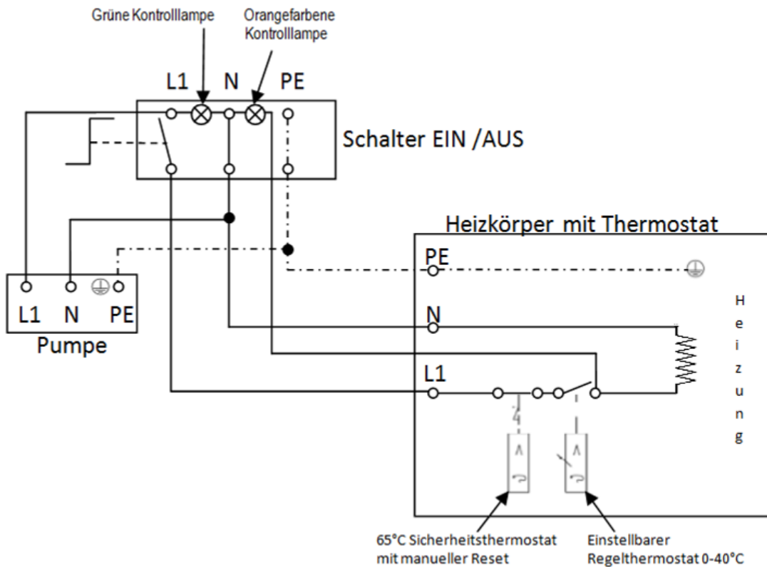
Aqualine mit Steuerung
