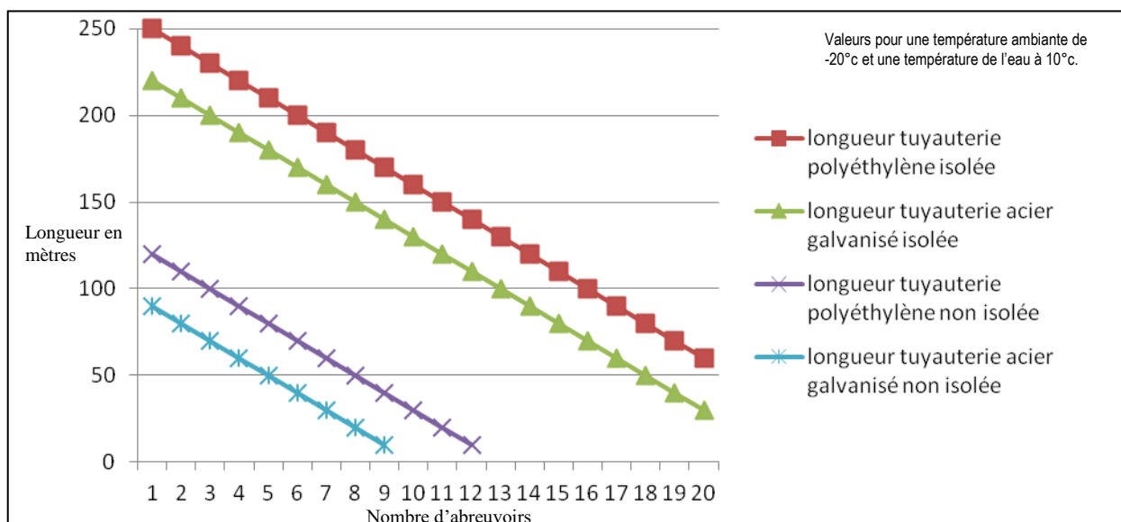
Diagramme 1 : Longueur maximale pour une tuyauterie en 3/4" ou 20 mm de diamètre intérieure
