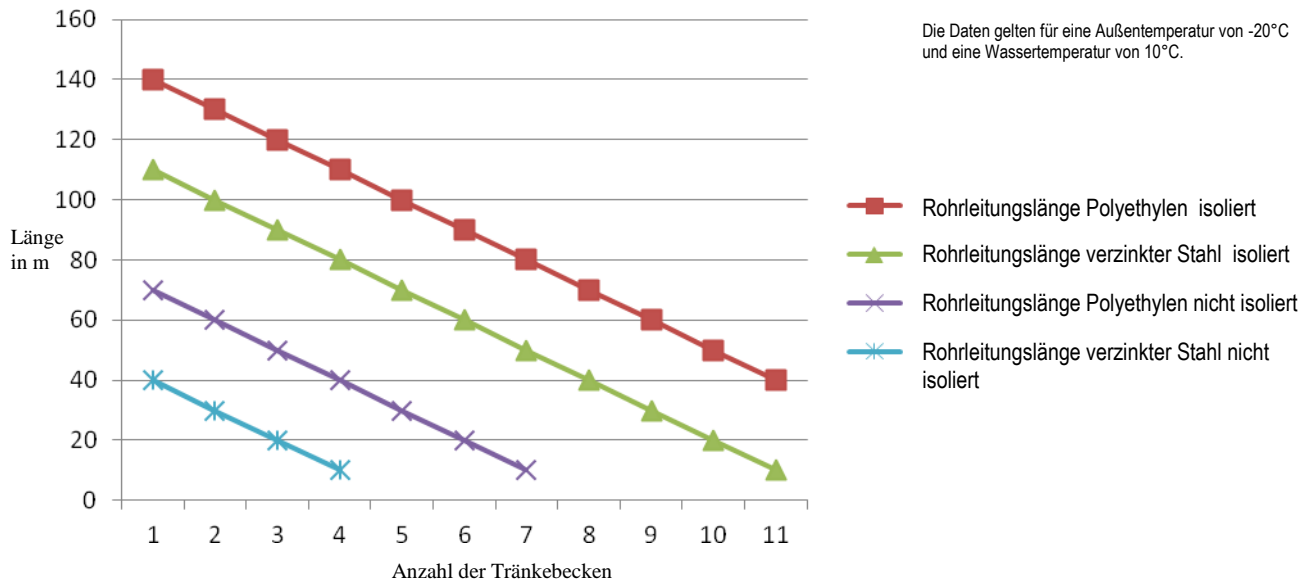
Diagramm 2: Maximale Länge für 1/2" Schlauch oder 15 mm Innendurchmesser
