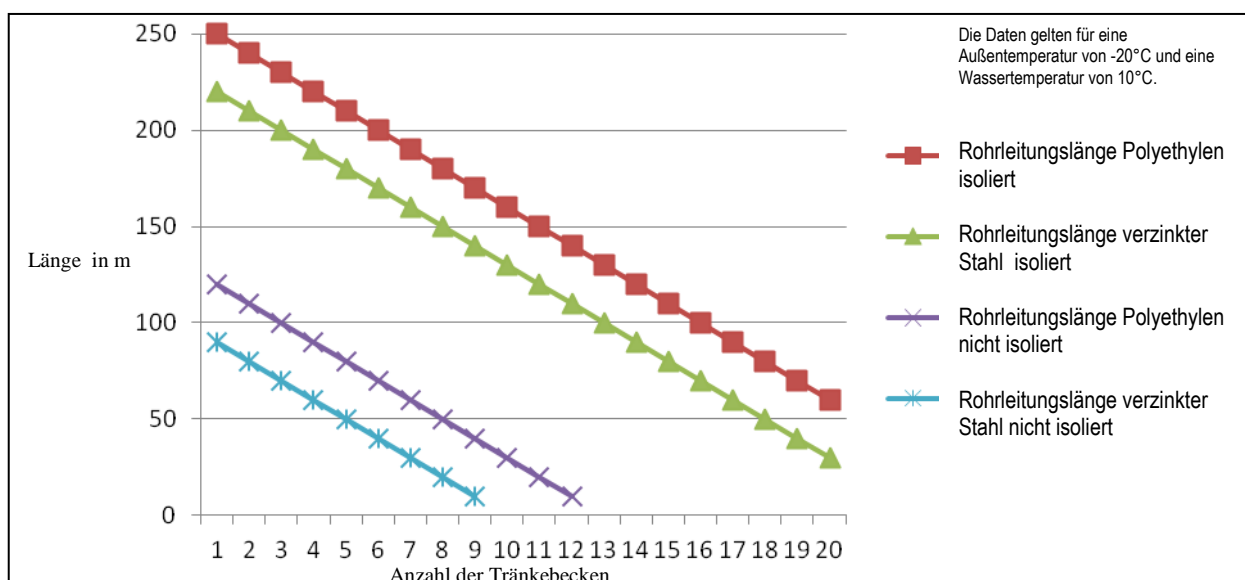
Diagramm 1: Maximale Länge für 3/4" Schlauch oder 20 mm Innendurchmesser
