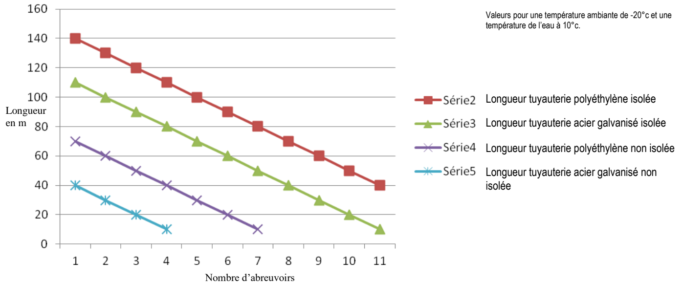
Diagramme 2 : Longueur maximale pour une tuyauterie en 1/2" ou 15 mm de diamètre intérieure
