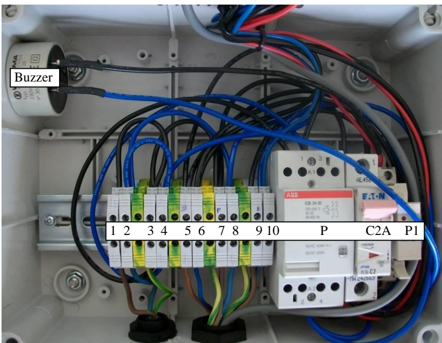
Photo intérieur boîtier contrôle digital
