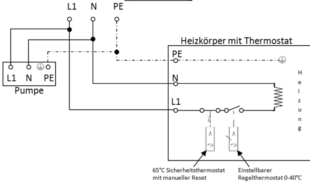
Aqualine ohne Steuerung
